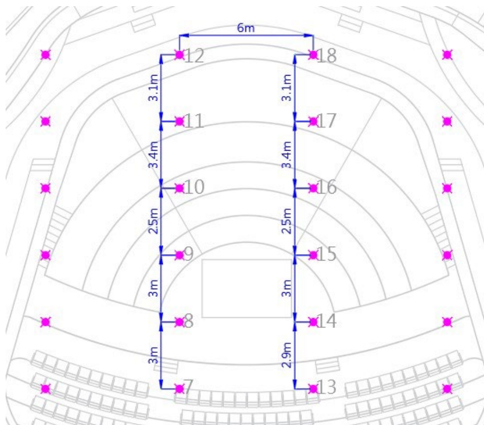
圖例 2.5.4 可放迴路鍊條馬達出線孔
