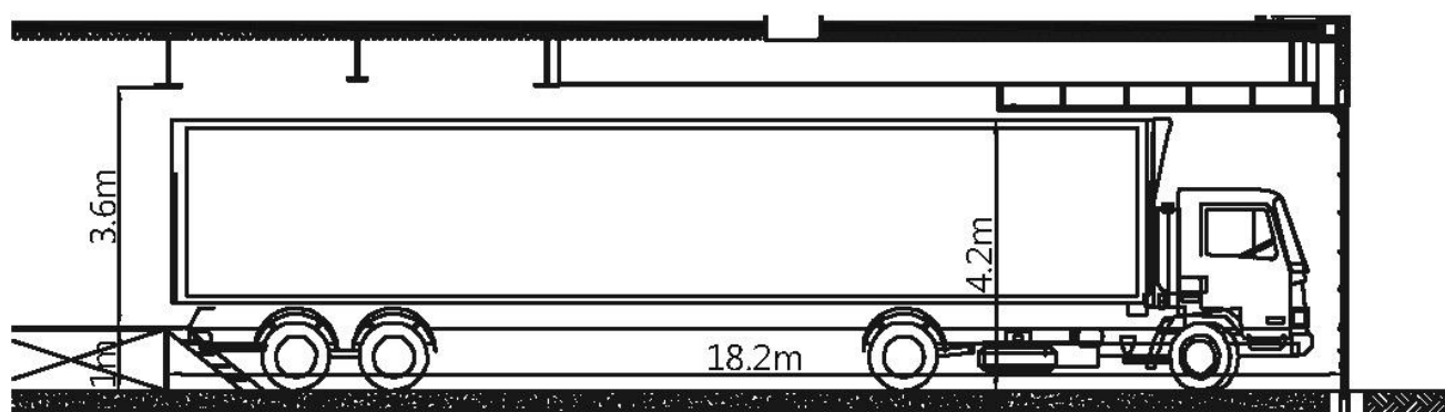
圖例 4.2 東碼頭卸貨口剖面圖
