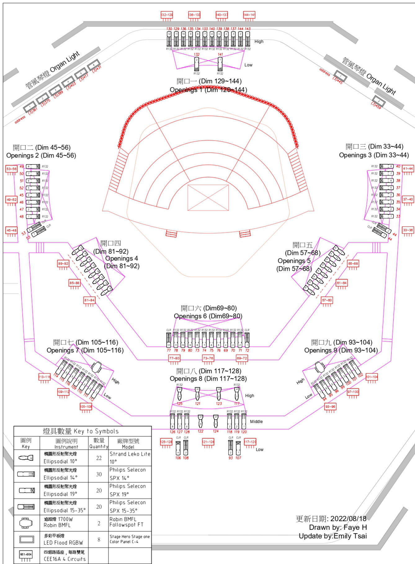
圖例 2.4.1 燈光基本配置圖
