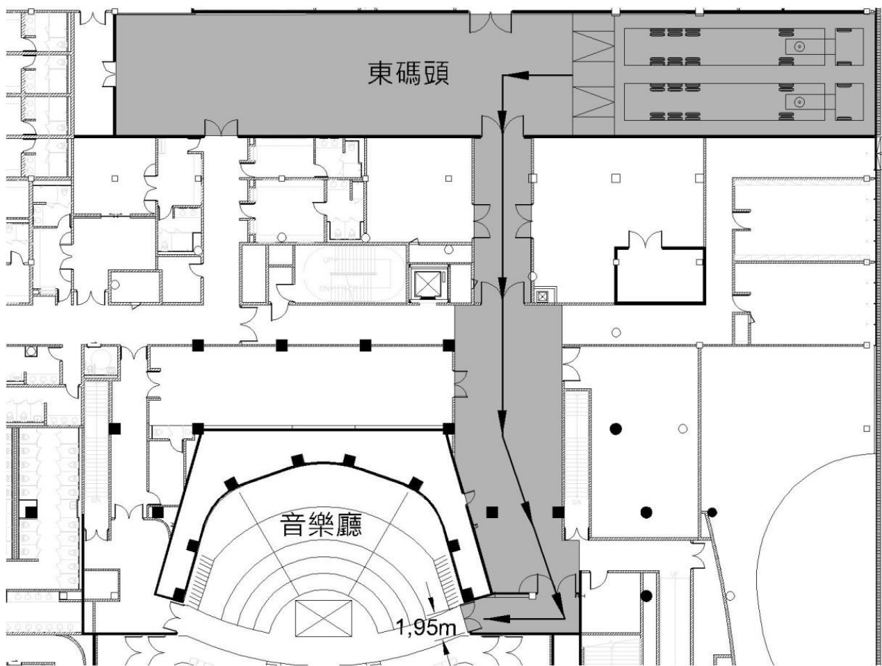
圖例 4.3 卸貨動線
