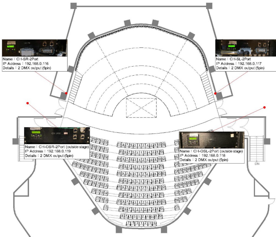
舞台區 Node 位置圖
