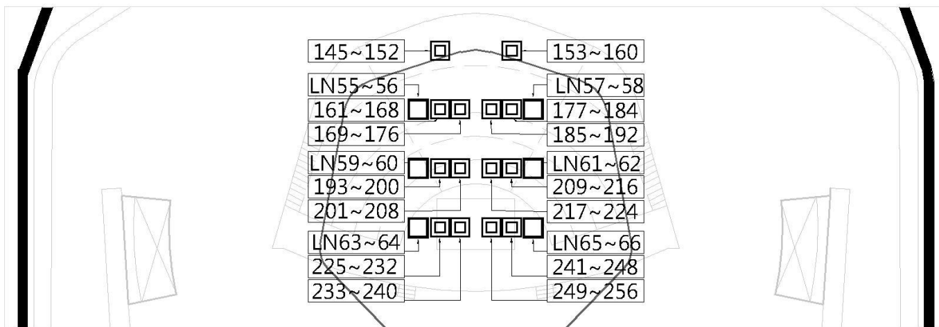
圖例 2.5.2 舞台頂棚區燈光迴路配置
