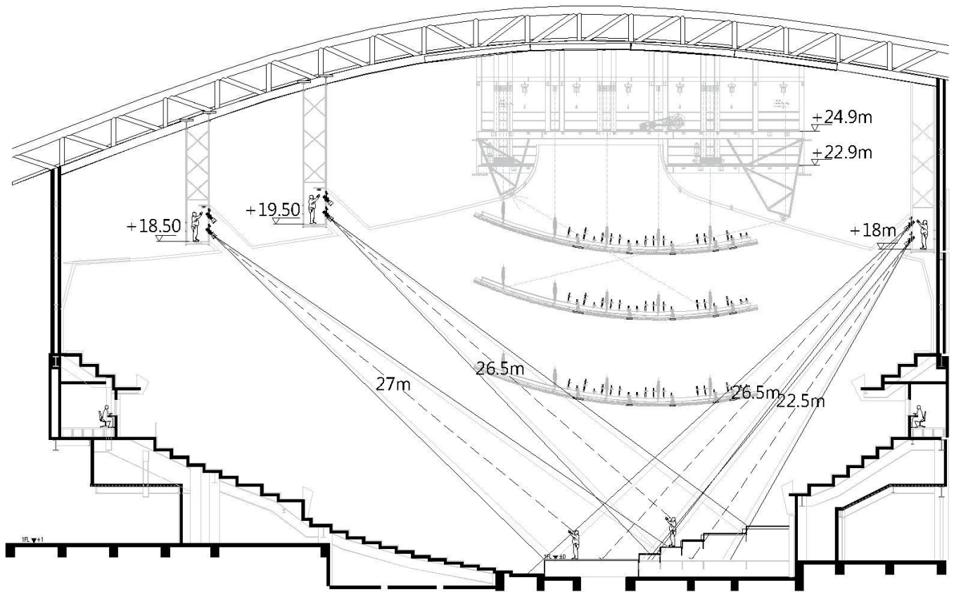
圖例 2.4.2 燈光剖面圖
