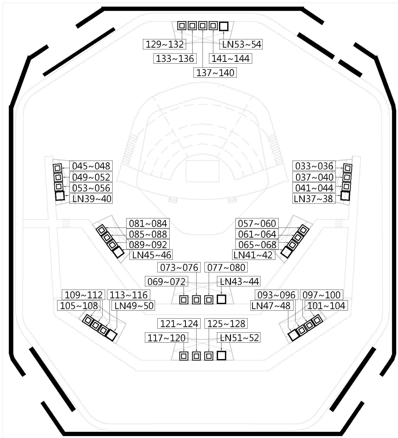
圖例 2.5.3 外區燈光迴路配置
